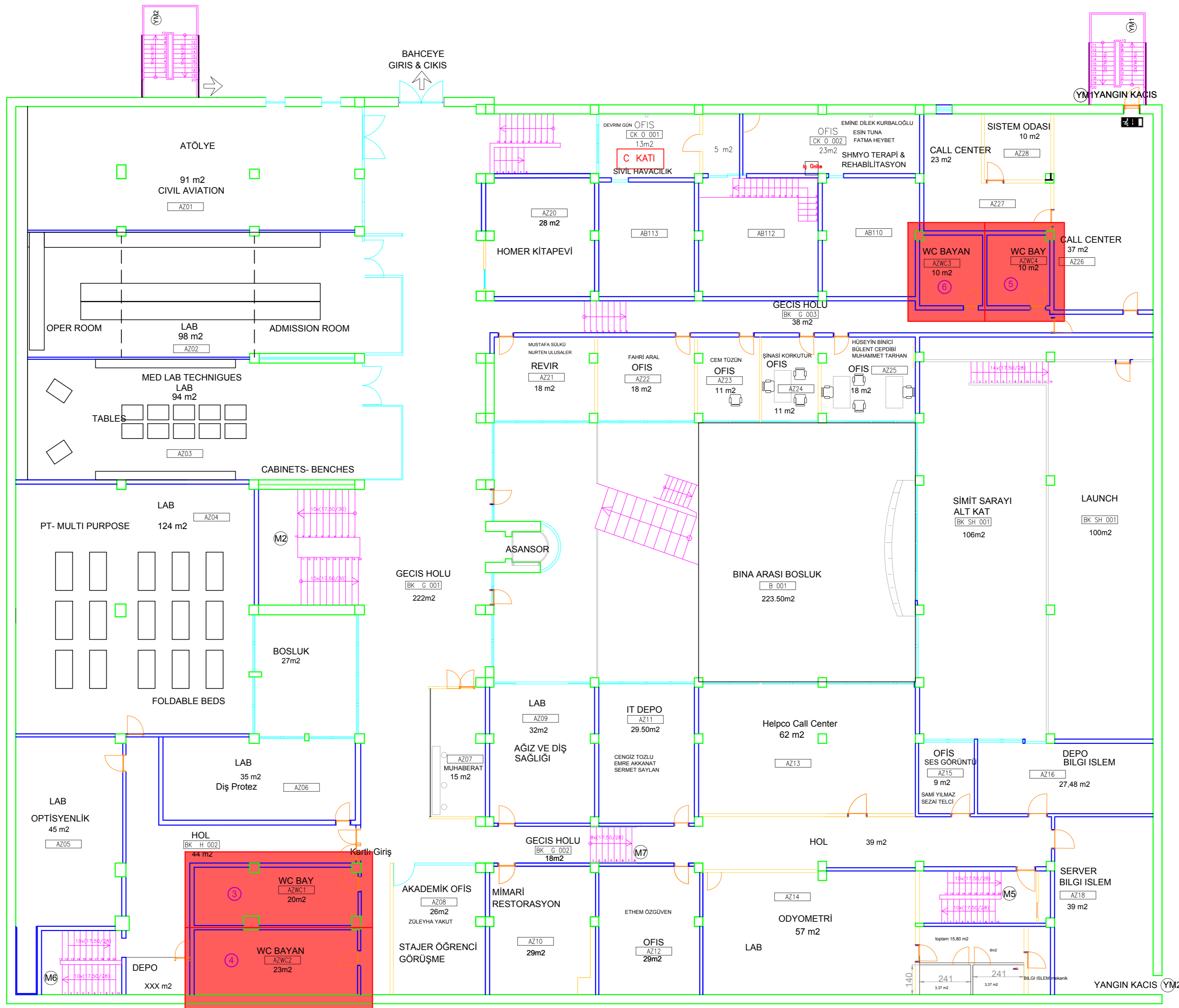
A BLOK ZEMİN KAT PLANI (ESKİ BİNA)
