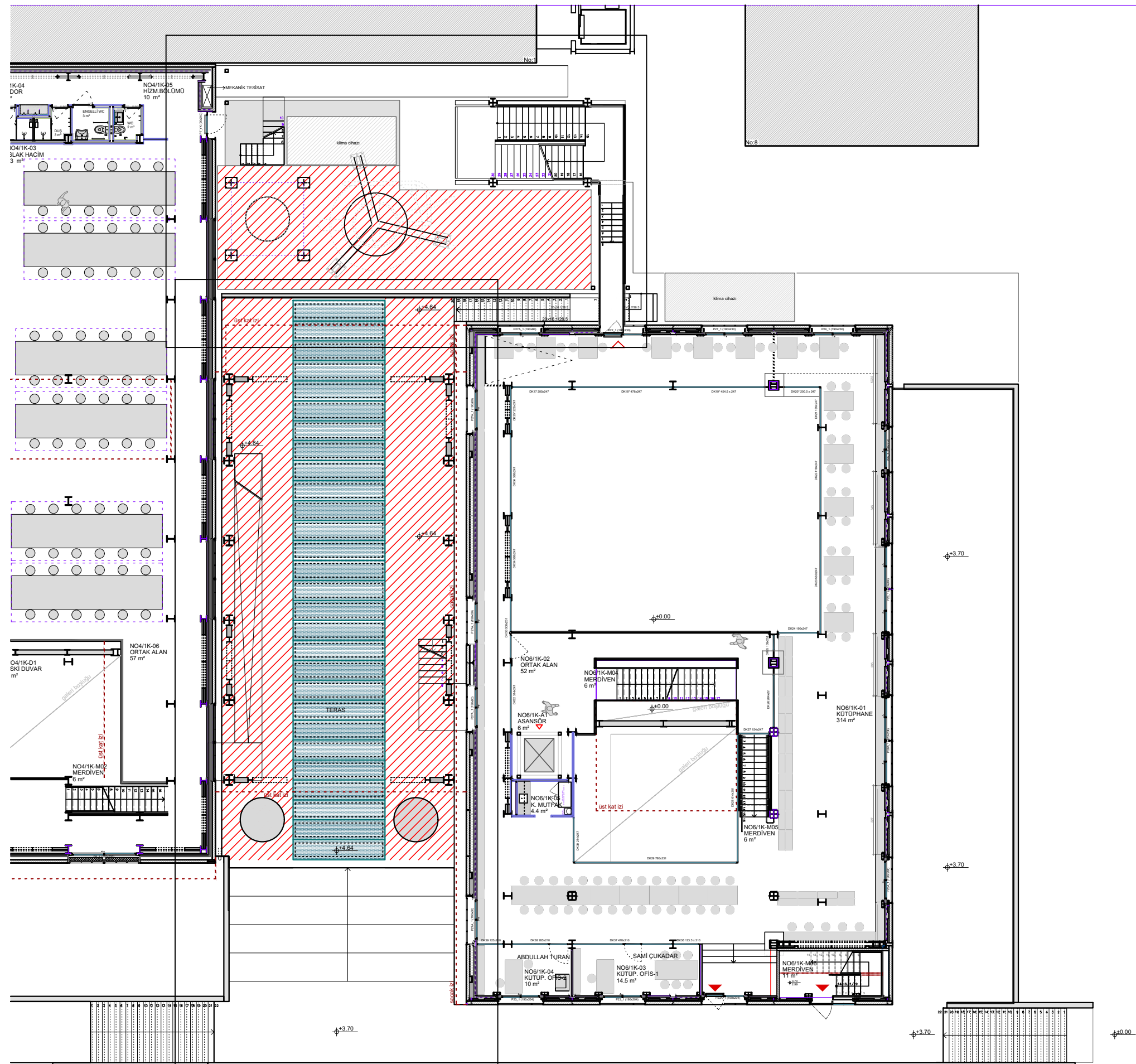
MİMARLIK CNC ATÖLYESİ – KÜTÜPHANE ÜSTÜ ÇATI PLANI
