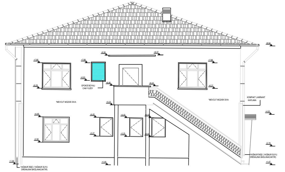
REKTÖRLÜK ÇATI GÖRÜNÜŞÜ
